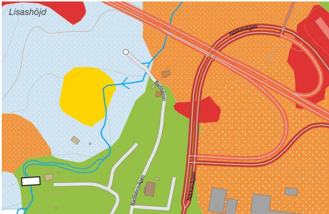
Utdrag från SGUs jordartskarta, grönt – isälvssediment, rött – urberg och orange – postglacial sand.
