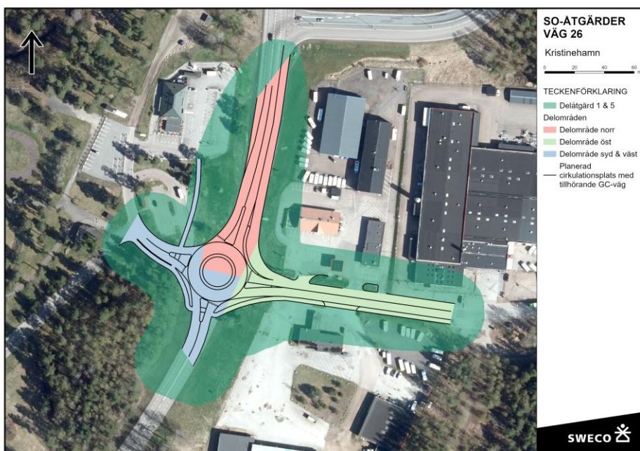
Figur 5-1. Delområden inom Delåtgärd 1 & 5 som använts för vidare beräkningar och föreslagen dagvattenhantering (Ortofoto: Lantmäteriet, geodatasamverkan. Cirkulationsplats och GC-väg: ritning 0201, Sweco, 2023b).
