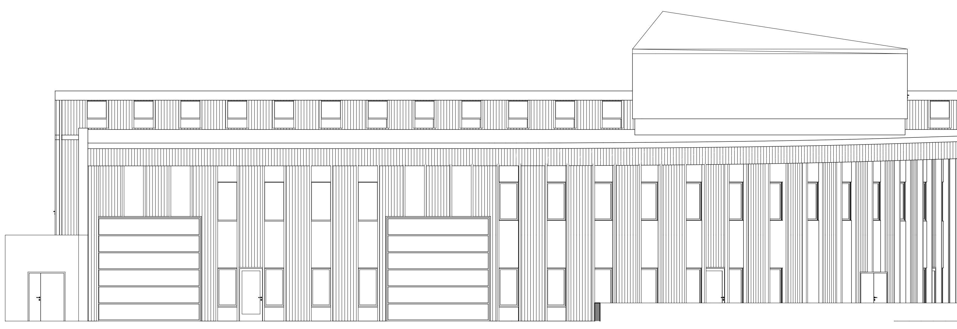
FASAD MOT VÄSTER A 1:100
